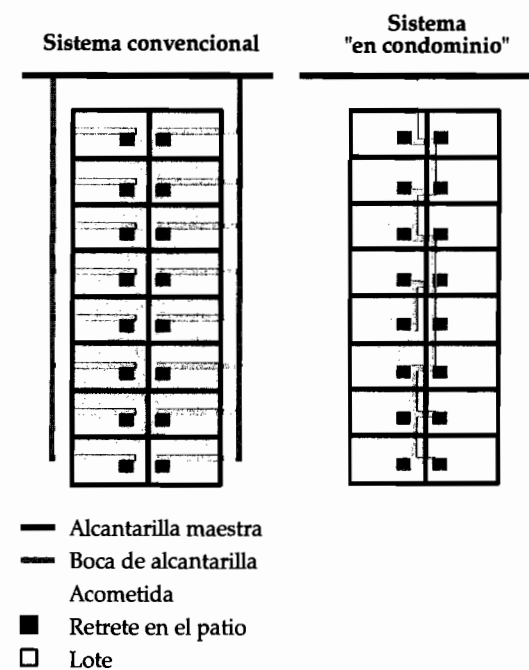
Figura R-5.5 Sistemas de alcantarillado convencionales y "en condominio"
